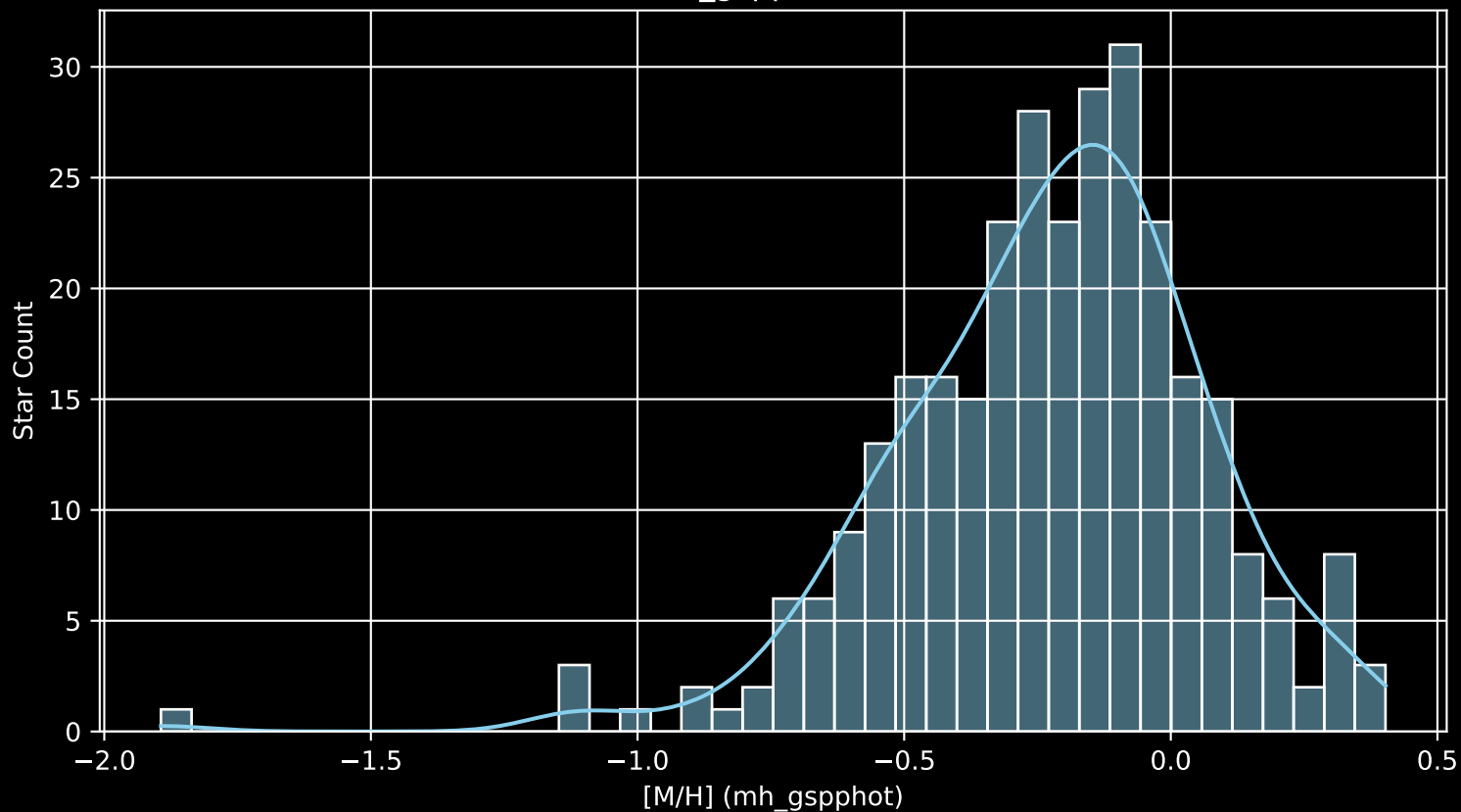
GALAH DR4 Field: [201] [M/H] (mh_gspphot) (n= 306)
