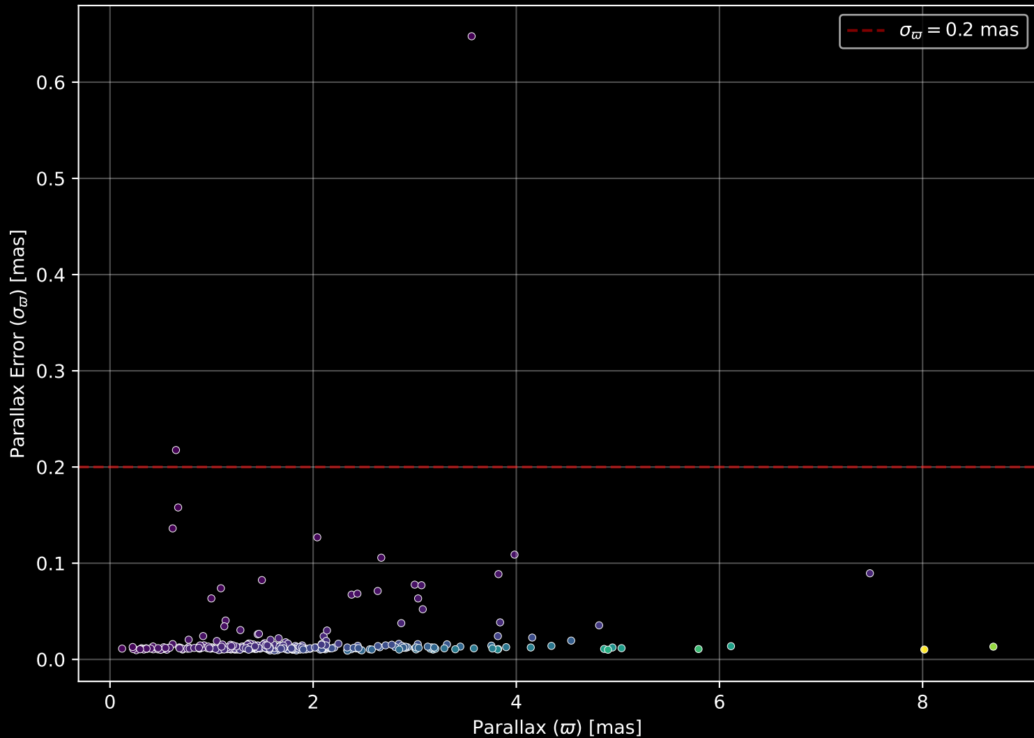
GALAH DR4 Field: [201] Parallax Quality (n= 307)
