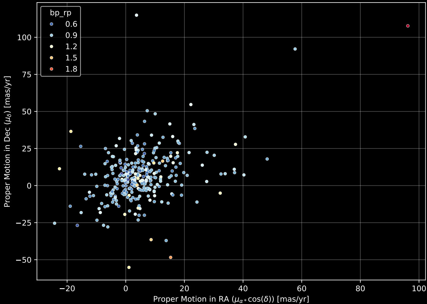
GALAH DR4 Field: [201] Proper Motion Diagram (n= 307)
