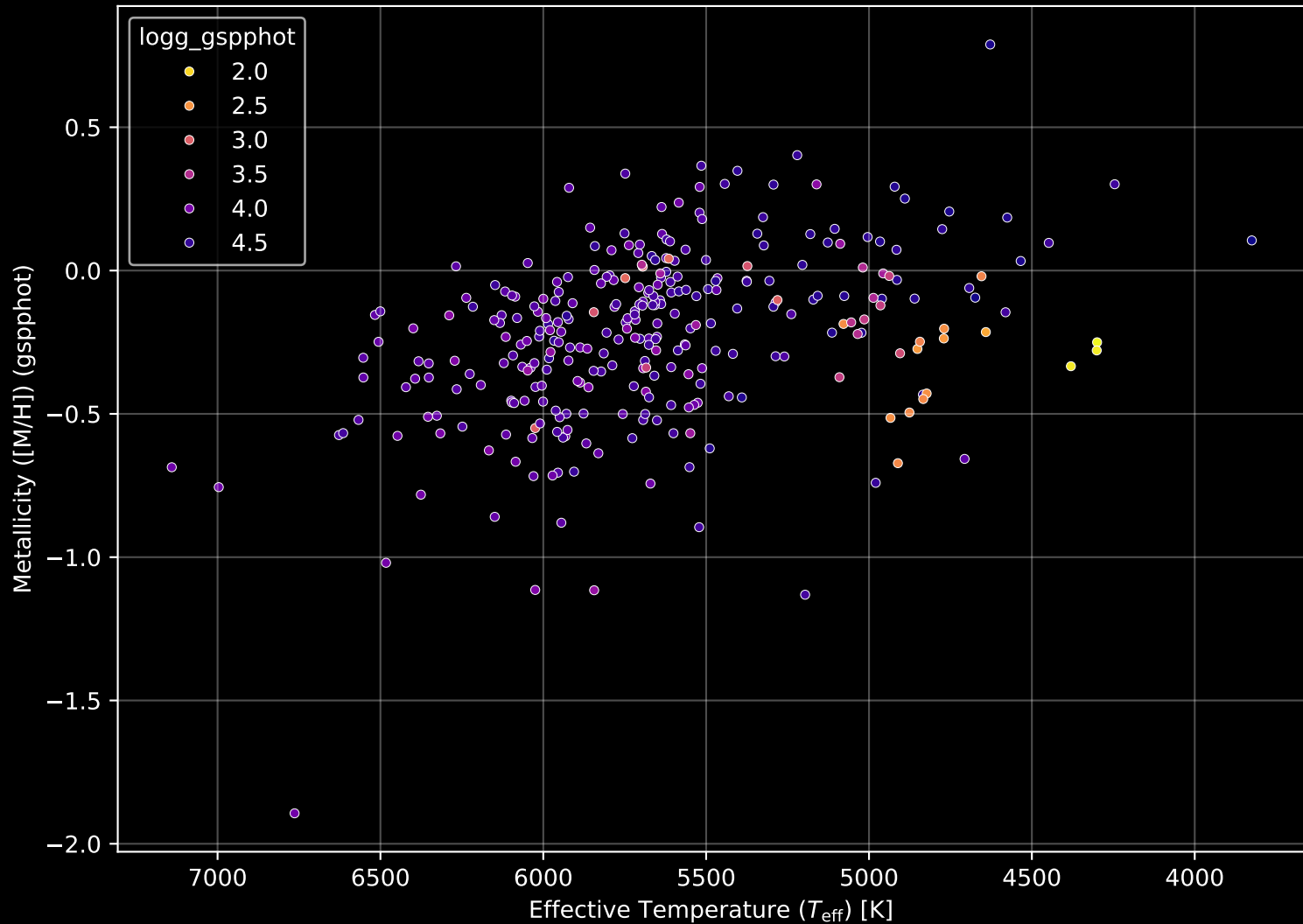
GALAH DR4 Field: [201] Stellar Population Parameters (n= 307)
